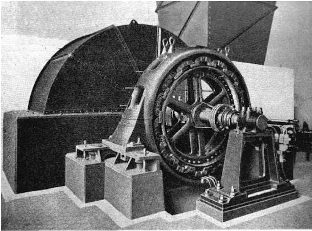
VENTILÁTOR S VODOROVNOU OSOU A ELEKTRICKÝM POHONEM VZOR VITKOVICKÝCH ZELEZAREN
